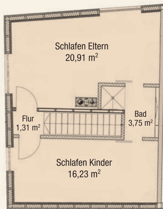
Obergeschoss
